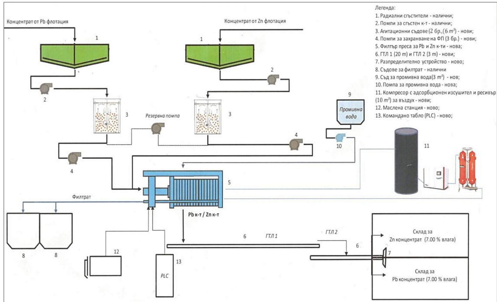
Слика 1 Нов систем за филтрирање на концентрати на Рb и Zn
